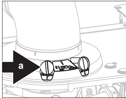
a Messpunkt Abgassonde Bild 15.1.a
