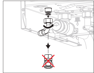
MAG-Set Membranausdehnungsgefäß Bild 8.2.a
