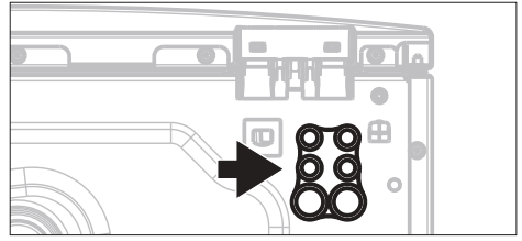
Kabeldurchführung an der Unterseite des Kessels
