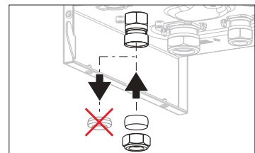
Membranausdehnungsgefäßanschluss Bild 8.2.b
