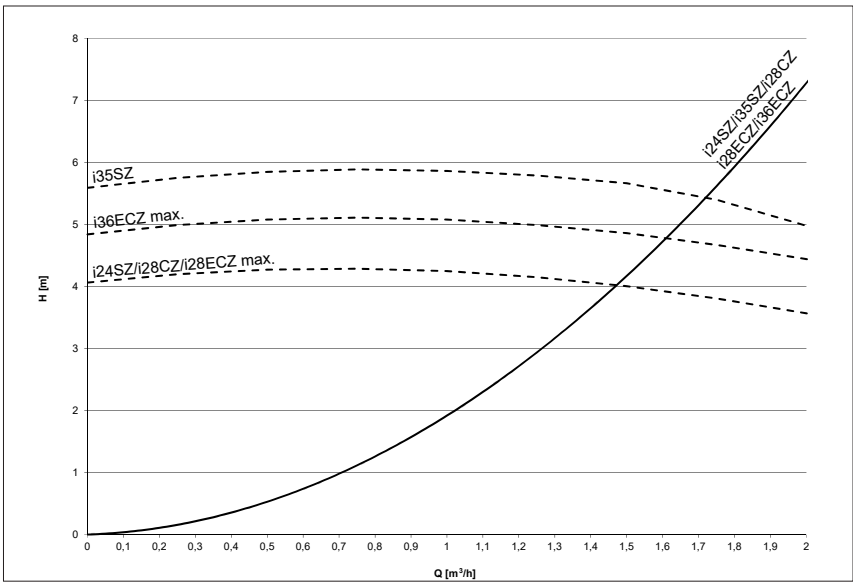
Pumpenkennlinien
