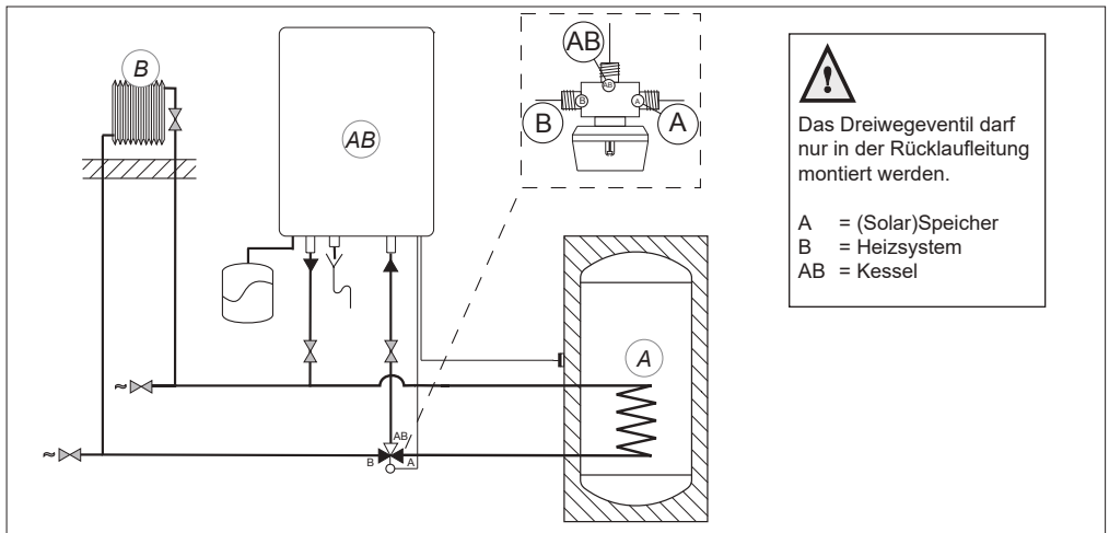
ATAG i24SZ oder i35SZ mit externem Speicher
