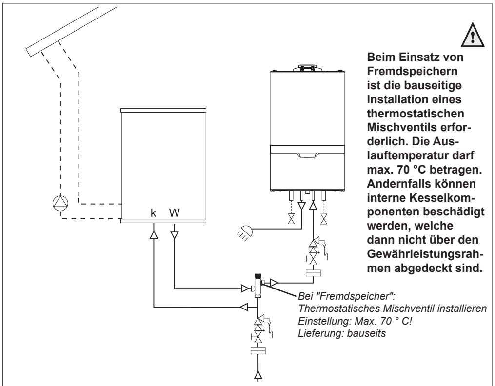
ATAG Kombikessel mit Solarspeicher
